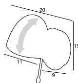
SG-623WRE 1x33W G9 230V (ze ściemniaczem / with dimmer)
