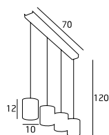
P0314-04B 4x20W G4 230V
