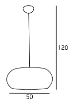
3826PB BK 3x60W E27 230V
