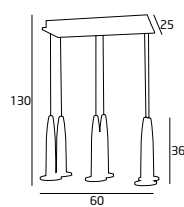
A6822-6 6x20W G4 230V
