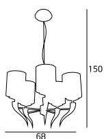
P0030 5x40W E14 230V
