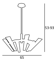
147 06 12 01 6x40W G9 230V
