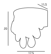
W0063 3x20W G4 230V
