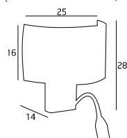
W0049 1x40W E27 230V (z włącznikiem / with switch)
