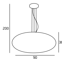
P10905-90B 3x60W E27 230V
