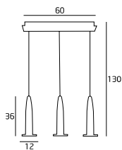
A6822-3X 3x20W G4 230V
