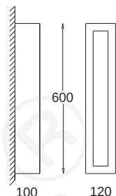
E27, 2 x max 23W LW 802g 7641
