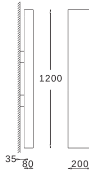
E27, 4 x max 23W LW 804g 7554
