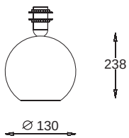
wersja mała / small version
