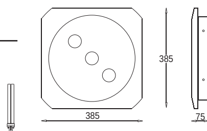
OB 330g 3815 magnetic ballast
