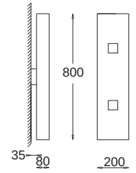
E27, 2 x max 23W LW 802g 7562
