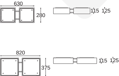
Calypso due plafon - wersja średnia / ceiling lamp - medium
