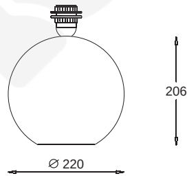
wersja duża / large version
